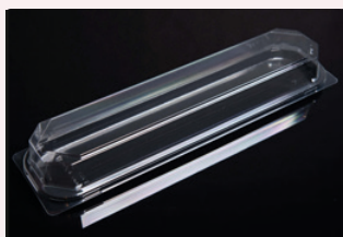
Lid 6A 1990 L: 407 x W: 107 x H: 15 mm
